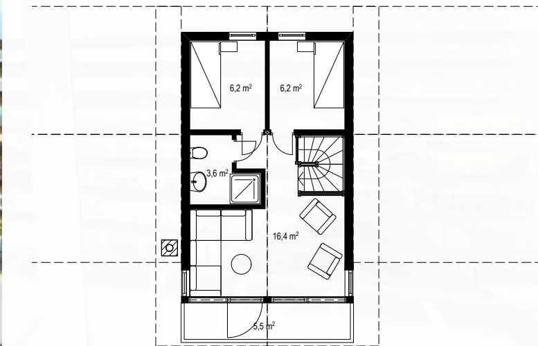
2. Floor 32,4 m 2
