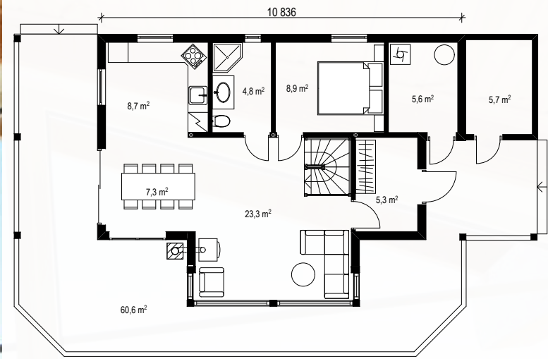
1. Floor 69,6 m 2
