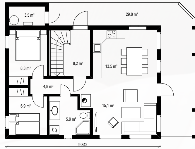
1. Floor 66,3 m 2
